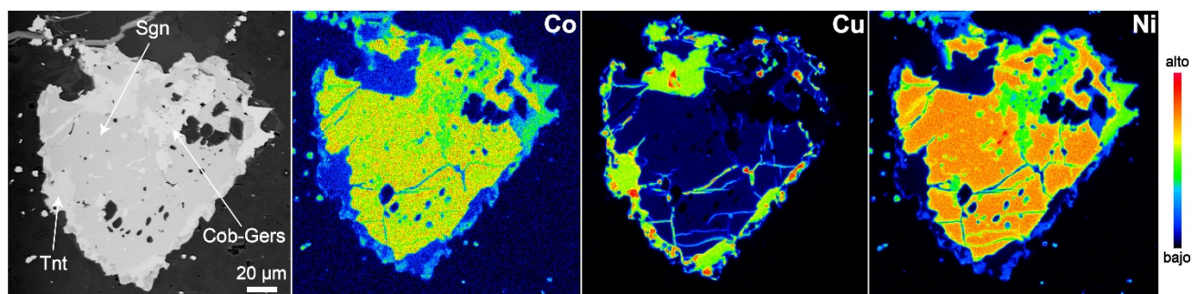
Fig 1. Cristal subhedral de siegenita (Sgn) y cobaltita-gersdorfit (Cob-Gers) con bordes de tennantita (Tnt).
