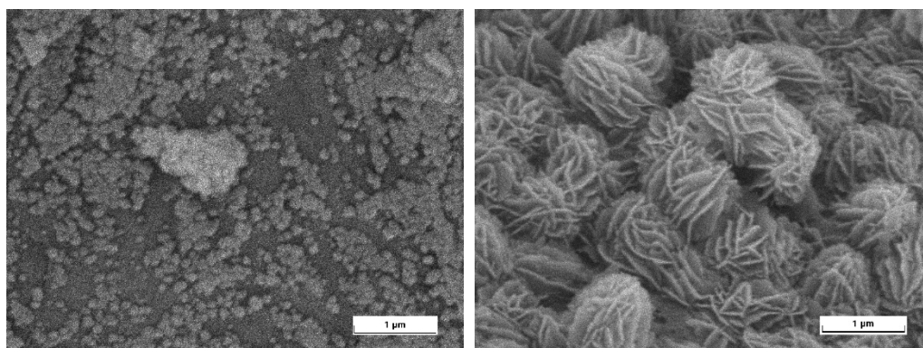
Fig 1. Imágenes de electrones retrodispersados de la superficie de fragmentos de jibia de sepia (Ar) (imagen izquierda) mostrando precipitados romboédricos de otavita, y fragmentos de jibia de sepia modificados (HAp) mostrando agregados de hidroxiapatito tapizando toda la superficie (imagen derecha). Ambas imágenes corresponden a la interacción de 50 ppm de \text{Cd}^{2+} durante 6 horas.
