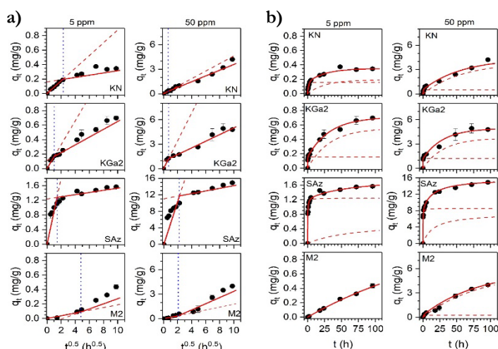
Fig. 1. a) Ajuste lineal del modelo IP modificado de la cinética de adsorción de TC sobre filosilicatos, b). Ajuste cinético en dos etapas de los modelos cinéticos de reacción en la adsorción de TC sobre filosilicatos. Las líneas discontinuas indica el ajuste a un modelo de adsorción individual y la línea sólida indica la suma de los dos modelos.
