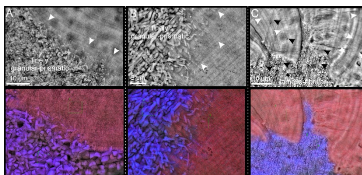
Fig 3. Imágenes de SEM (A-C) y sus respectivos mapas de EDX ( Mg^{2+} en color azul) de diferentes esférulitos de aragonito sustituyendo a la calcita granular-prismática en Spirobranchus giganteus .
