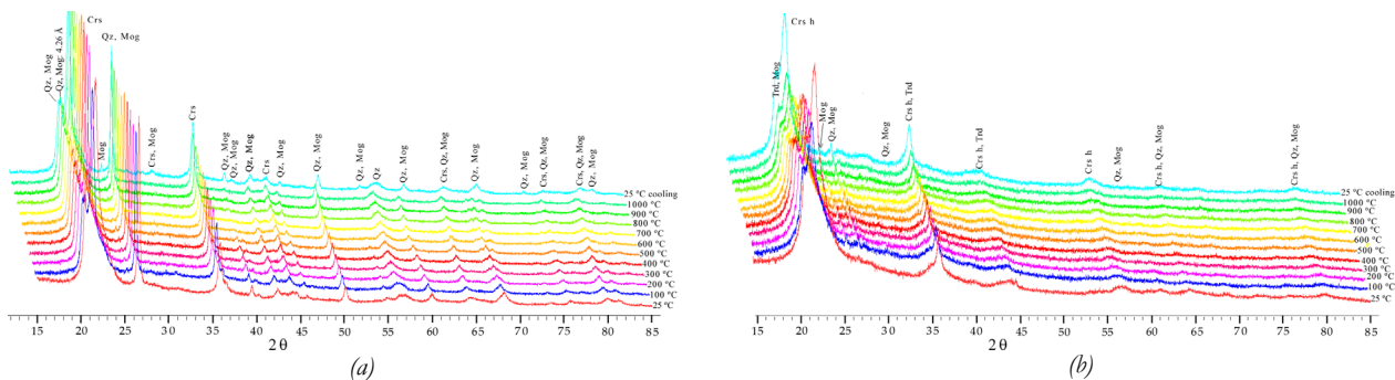
Fig. 2 Diagramas DRX del tratamiento térmico in situ: (a) Cerro Almodóvar, (b) La Marañosa.
