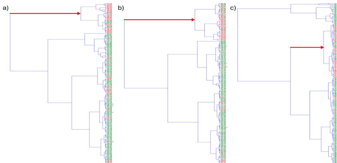
Fig 1. a) Cluster obtenido con el valor de 816 nm en la primera derivada. b) Cluster multivariado con el valor de 806 nm en la primera derivada. c) Cluster multivariado con el valor de 805 nm en el continuum removal . Rojo: muestras > 400 ppm U_3O_8 ; Verde: muestras < 400 ppm U_3O_8 .
