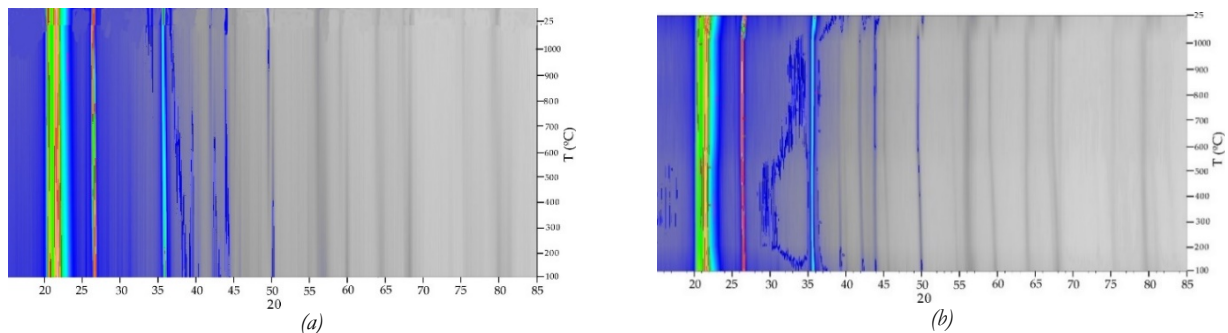
Fig. 3 Diagramas DRX 2D de falso color del tratamiento térmico in situ: (a) Cerro Almodóvar, (b) La Marañosa.
