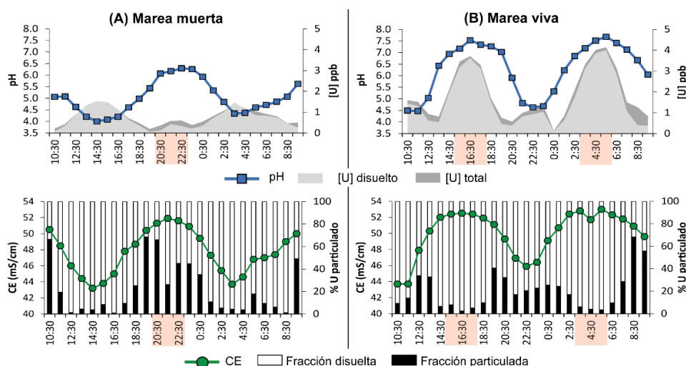
Fig 1. Evolución del pH, CE, concentración total y disuelta de U y fracción de U en el material particulado en (A) fase de marea muerta y (B) fase de marea viva en ciclos de marea. Sombreado en rojo se destacan las pleamareas.
