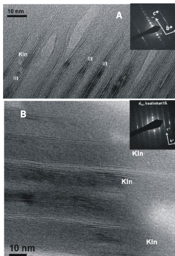
Figura 4. A. Imagen HRTEM de la matriz de las rocas en la que se muestra que la caolinita (Kln) está interestratificada con capas de illita (Ill). En el recuadro superior derecho se muestra el patrón de difracción que refleja que estas arcillas tienen politipos desordenados. fig. 4B. Imagen HRTEM de la matriz de las rocas que muestra zonas ricas en caolinita (Kln) con defectos cristalinos como terminaciones de las capas y franjas reticulares onduladas. En el cuadrado superior derecho se observan el patrón de difracción que sugiere politipos desordenados. Kln=caolinita, Ill=illita.
