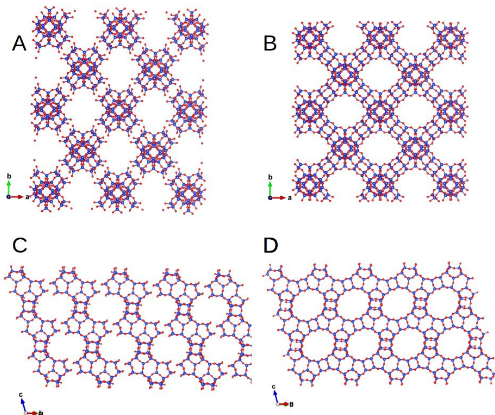
Fig.2. El silicato en cadena ZEO-2 (A y C) condensa topotácticamente al calcinar, dando lugar a la zeolita ZEO-3 con un sistema 3D de poros extragrandes (16 tetraedros, B, 14 tetraedros, D).
