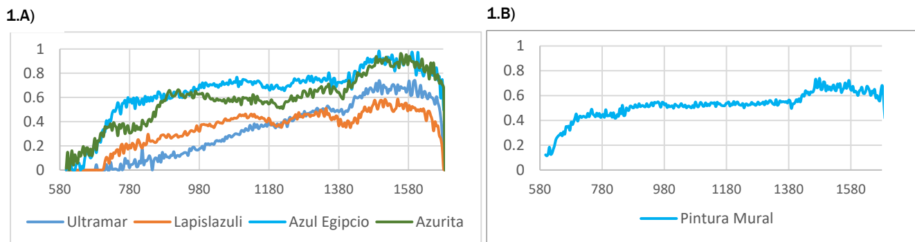
Figura 1: A) Firmas espectrales obtenidas a partir de los estudios de pigmentos en polvo: Ultramar Kremer 45010, Lapislázuli Kremer 10520, Azul Egipcio Kremer 10060 y Azurita Kremer 10200. B) Firma espectral pigmento Azul Egipcio en probeta de pintura mural.
