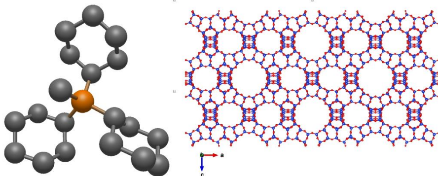
Fig.1. El catión \text{Cy}_3\text{MeP}^+ (Izquierda) dirige la cristalización de ZEO-1 la primera zeolita con un sistema 3D de poros extragrandes (y poros grandes) interconectados, claramente visibles en la imagen de la derecha. Azul Si o Al, rojo O, negro C, dorado P.
