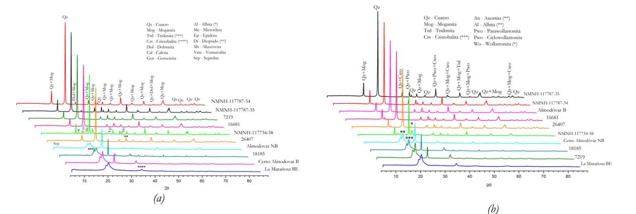
Fig. 1 Diagramas DRX de las muestras sin tratar (a) y las tratadas térmicamente ex situ (b).
