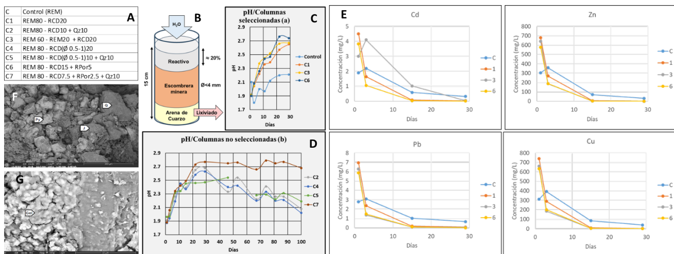
Fig 1. A. Composición de las columnas preparadas. B. Diseño de las columnas. C y D. Valores de pH de las columnas seleccionadas y no seleccionadas. E. Concentración de Cd, Cu, Pb y Zn en las columnas seleccionadas. F y G. Fotos de microscopía electrónica. F. Foto general con presencia de pirita, cuarzo y jarosita. G. Precipitados de geles de hierro y sílice ricos en Cu y Zn.
